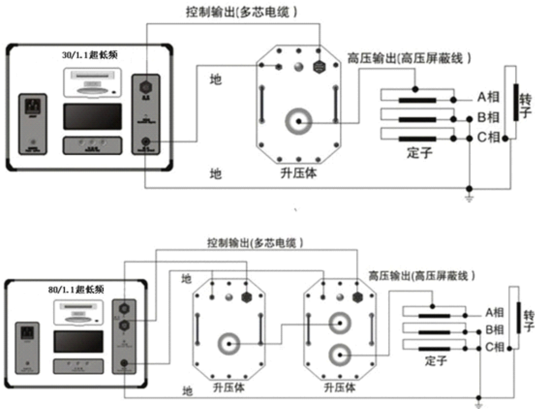
图18a/b 测量定子的某相连线图
