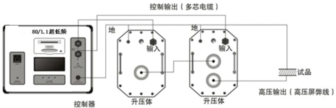
图 4b 80/1.1 (连线图)
